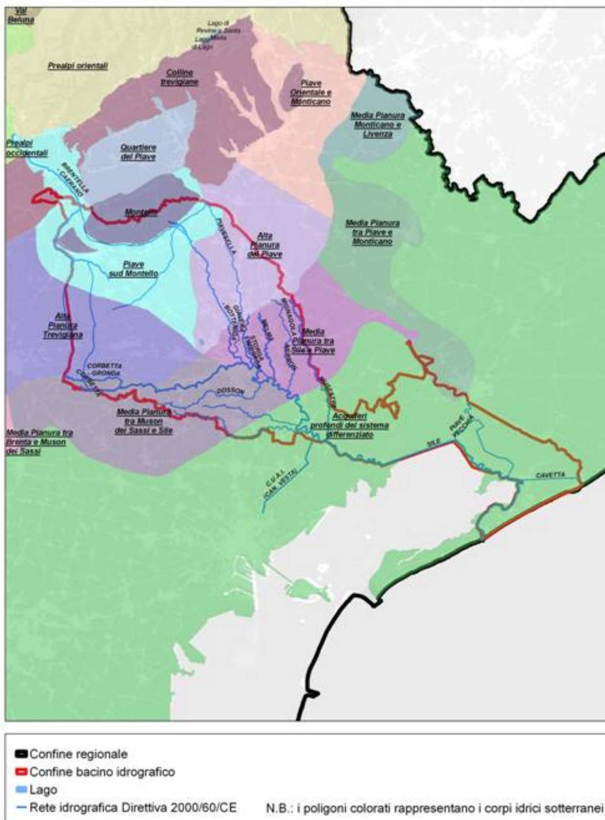
Figura 1.8: Corpi idrici sotterranei ricadenti nel bacino del Sile. Coincide con la carta dei bacini idrogeologici
